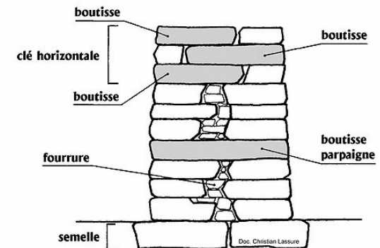
COUPE D'UN MUR EN PIERRE SECHE
